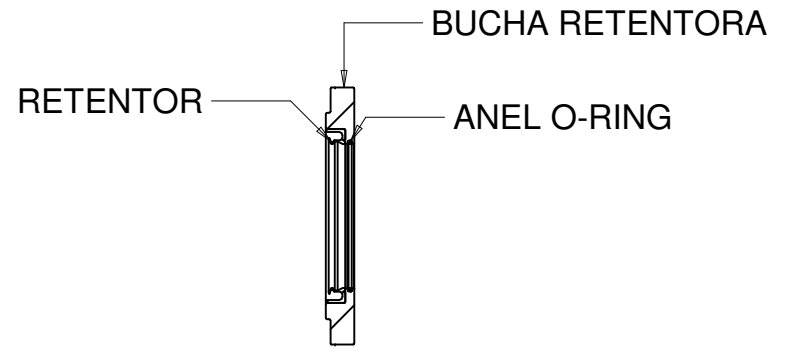
CONJUNTO BUCHA RETENTORA
